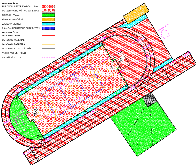
ilustrace technického výkresu mikulášovického atletického oválu a multifunkčního hřiště
